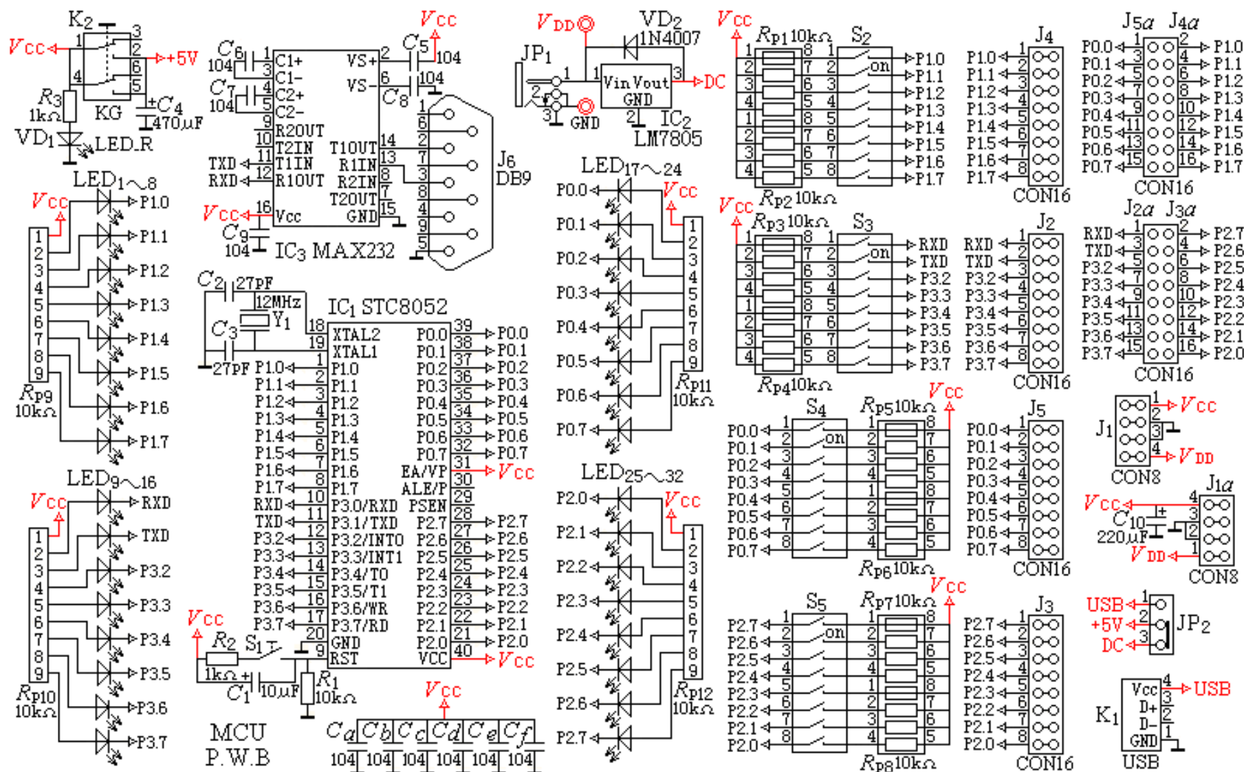
附图 2 主机控制电路图
